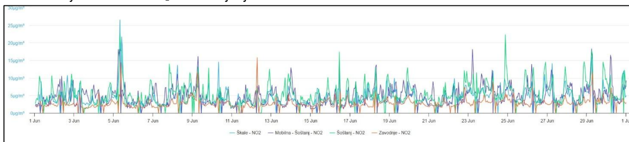
Graf 2: Izmerjene vrednosti NO 2 v mesecu juniju 2026
