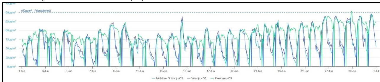
Graf 3: Izmerjene vrednosti O_3 v mesecu juniju 2026
