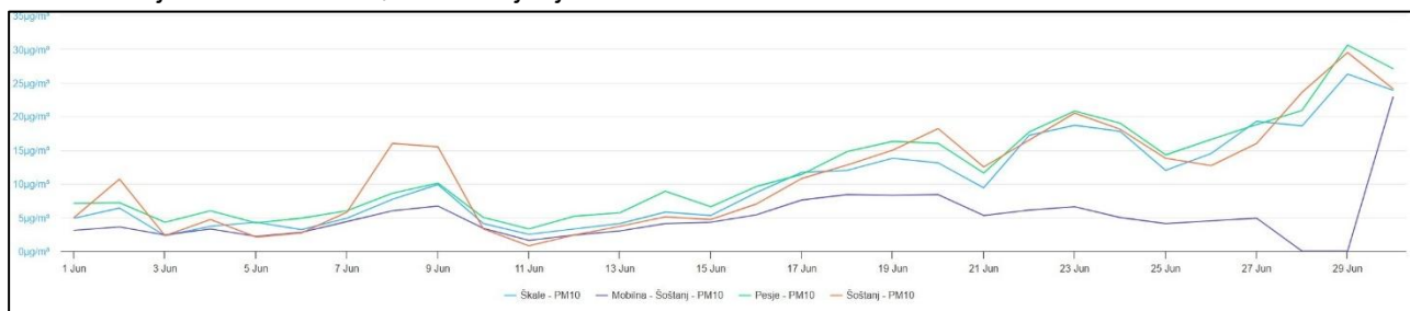
Graf 4: Izmerjene vrednosti PM_{10} v mesecu juniju 2026
