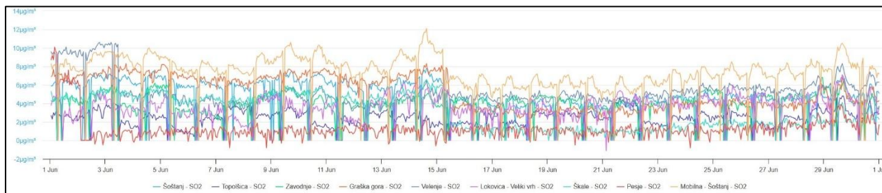
Graf 1: Izmerjene vrednosti SO 2 v mesecu juniju 2026
