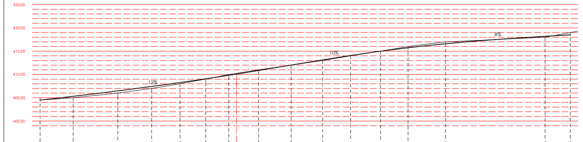
PROFIL P4 (cesta c2)
