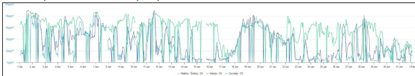
Graf 3: Izmerjene vrednosti O_3 v mesecu januarju 2026
