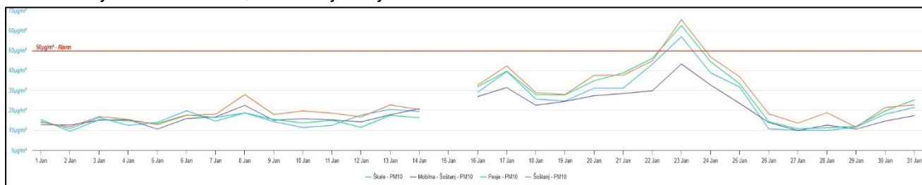
Graf 4: Izmerjene vrednosti PM_{10} v mesecu januarju 2026
