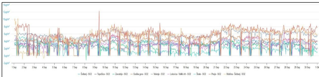
Graf 1: Izmerjene vrednosti SO 2 v mesecu septembru 2025
