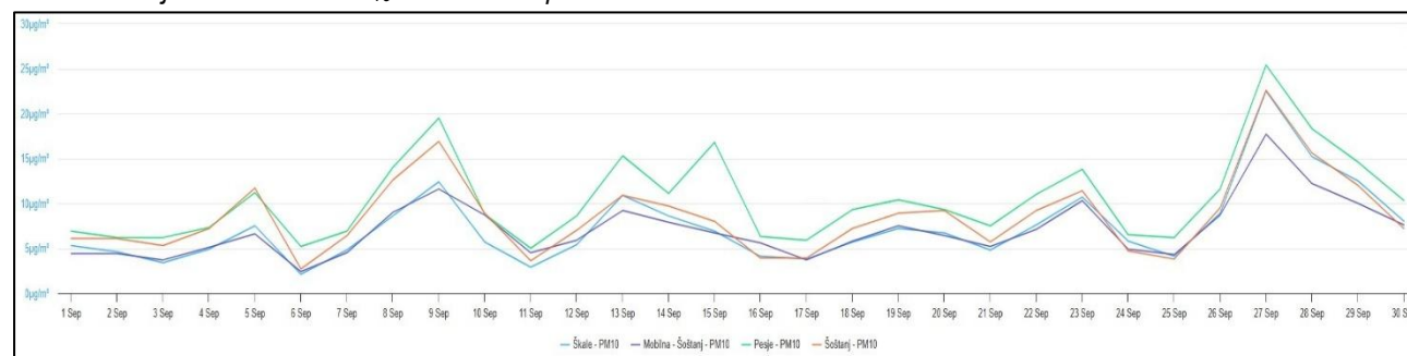
Graf 4: Izmerjene vrednosti PM_{10} v mesecu septembru 2025
