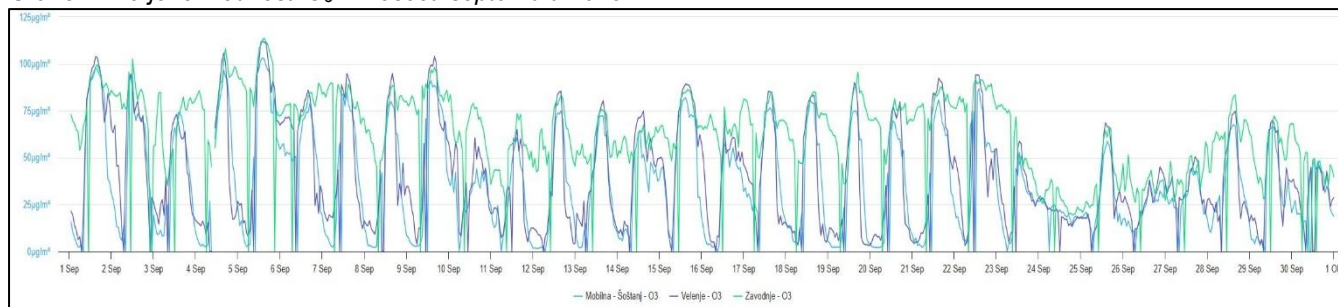
Graf 3: Izmerjene vrednosti O_3 v mesecu septembru 2025
