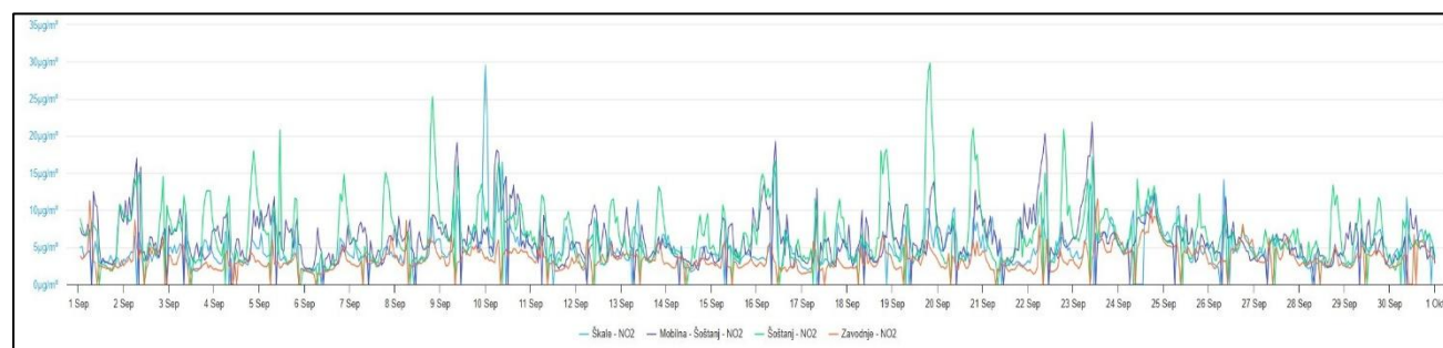
Graf 2: Izmerjene vrednosti NO 2 v mesecu septembru 2025
