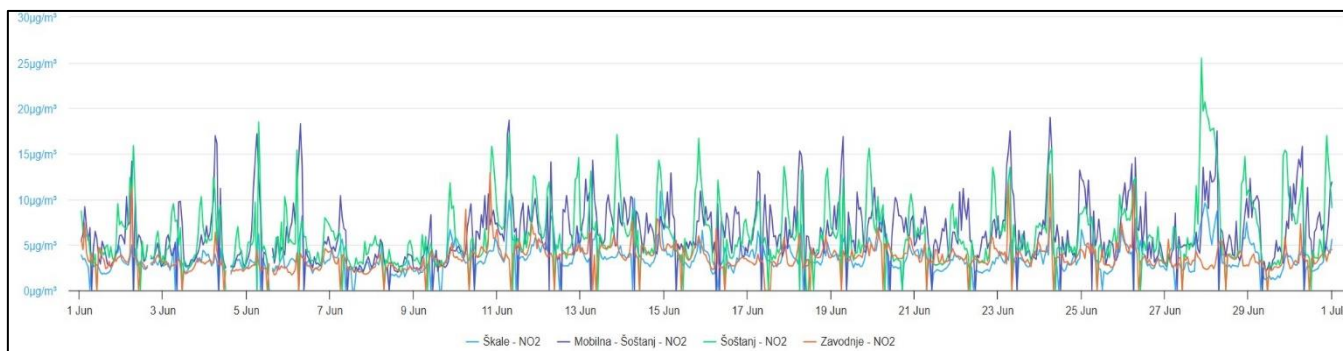
Graf 2: Izmerjene vrednosti NO 2 v mesecu juniju 2025
