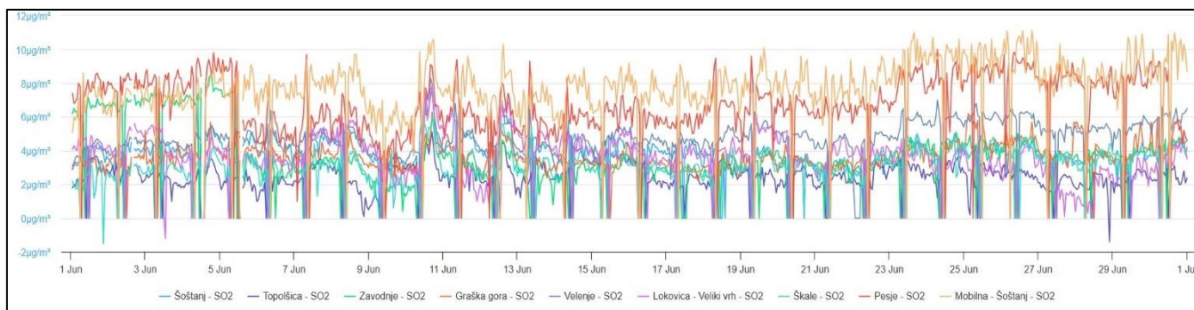
Graf 1: Izmerjene vrednosti SO 2 v mesecu juniju 2025
