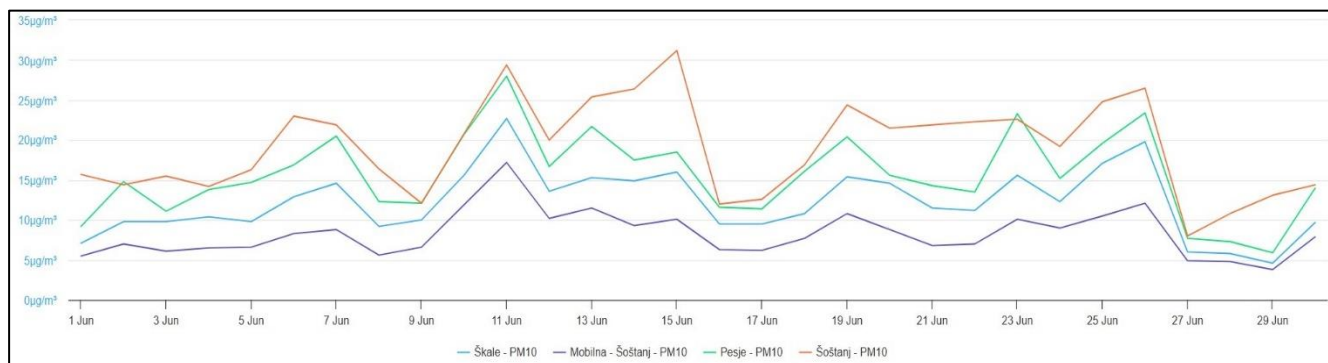
Graf 4: Izmerjene vrednosti PM_{10} v mesecu juniju 2025
