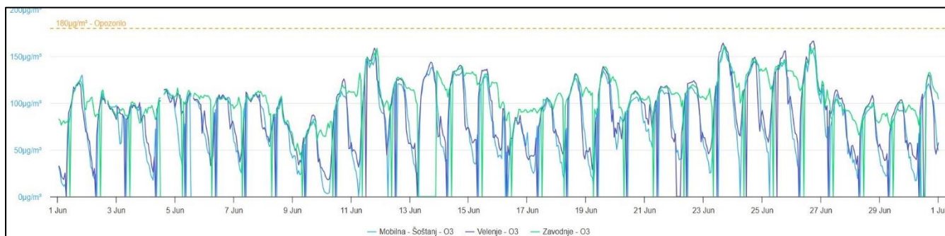
Graf 3: Izmerjene vrednosti O_3 v mesecu juniju 2025
