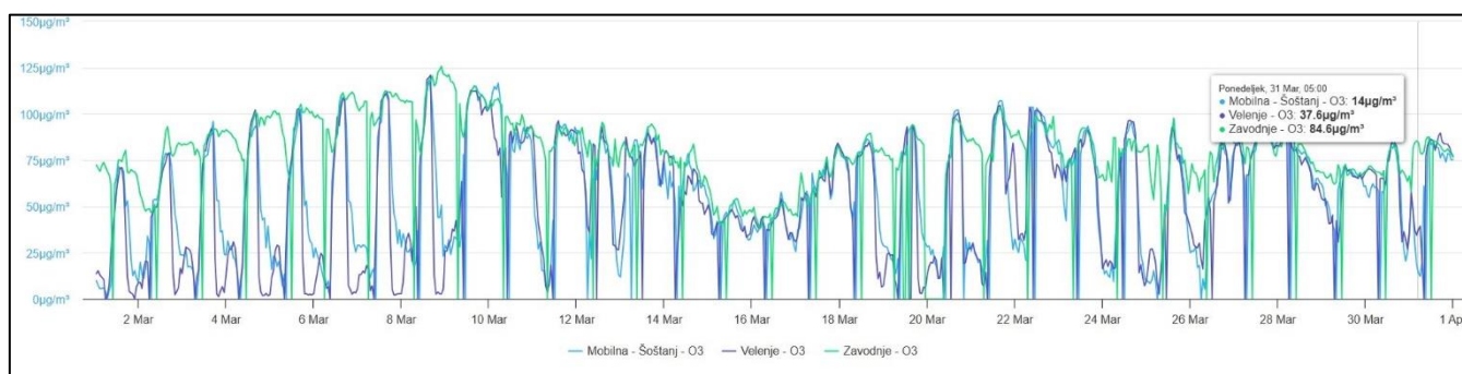
Graf 3: Izmerjene vrednosti O_3 v mesecu marcu 2025
