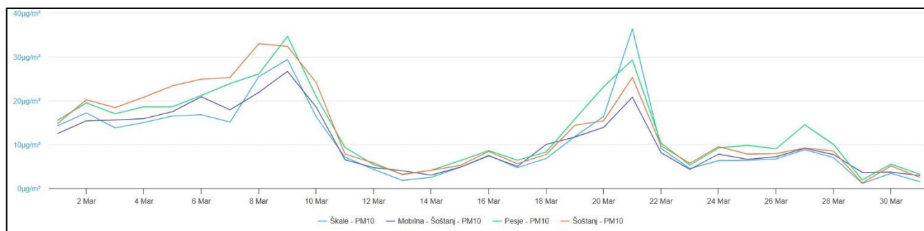
Graf 4: Izmerjene vrednosti PM_{10} v mesecu marcu 2025
