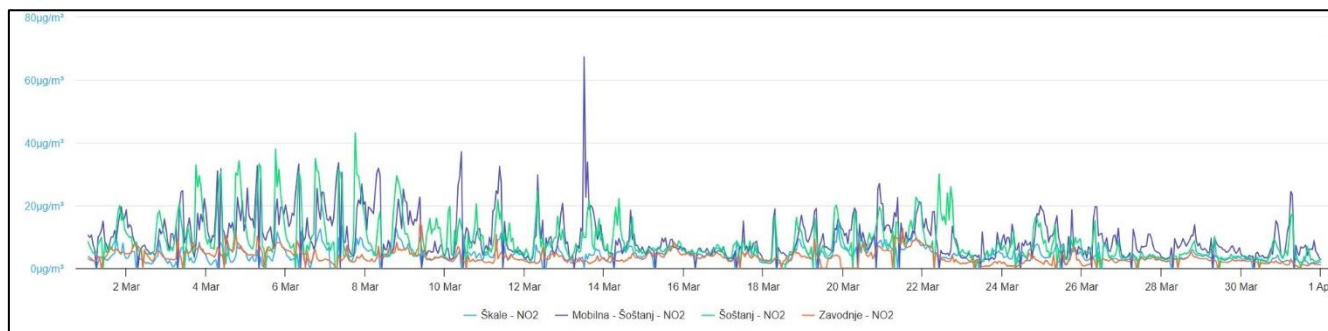
Graf 2: Izmerjene vrednosti NO 2 v mesecu marcu 2025
