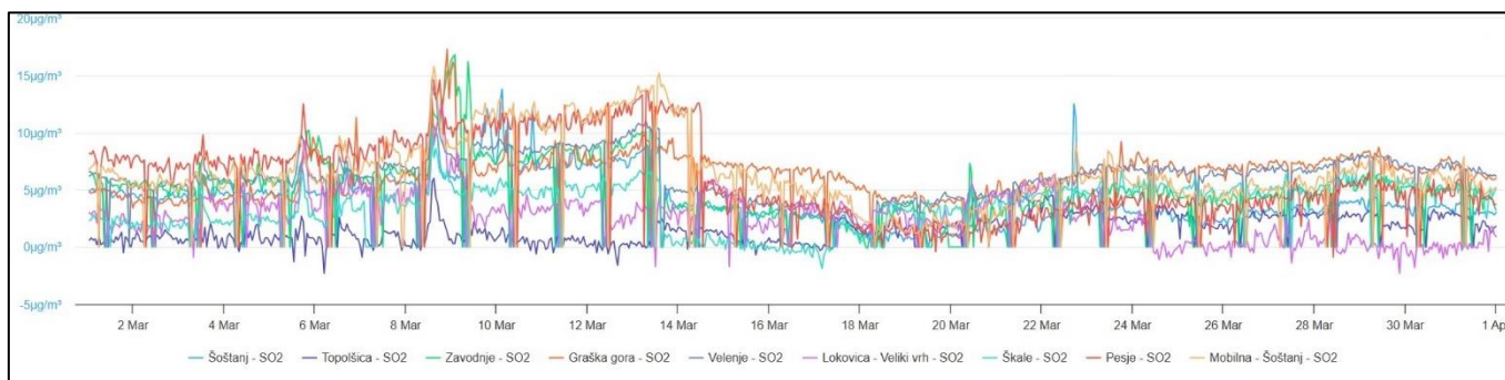
Graf 1: Izmerjene vrednosti SO 2 v mesecu marcu 2025
