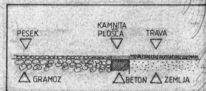
PEŠČENE POTI V PARKU - DETAIL STIKA
