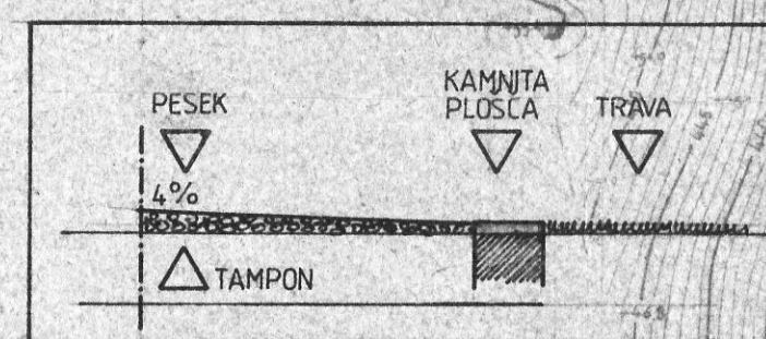
MAKADAMSKA URGENTNA CESTA SKOZI PARK - PREREZ
